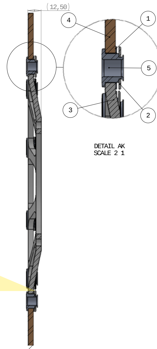
SECTION AJ-AJ
