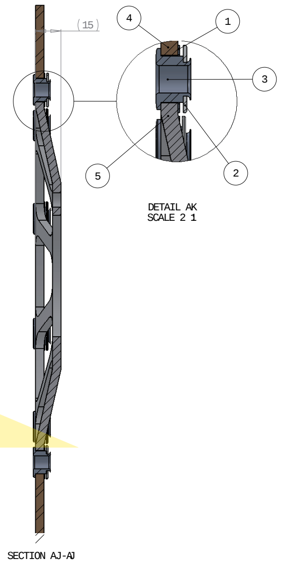
SECTION AJ-AJ
